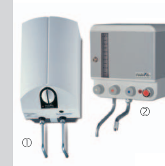
① Водонагреватель FKS 5 ② Водонагреватель FOKW 5 ① Hot Water Heater FKS 5 ② Water Heater FOKW 5
